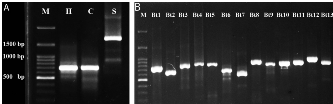
شکل ۲. A) قطعات ژنومی تکثیرشده جدایه ایرانی ویروس موزاییک چغندر در آزمون RT-PCR با استفاده از آغازگرهای دژنره Sprimer و M4T (چاهک S)، CIFor و CIRev (چاهک C) و HPFor و HPRev (چاهک H). M مارکر ۱۰۰ جفت‌بازی. B) قطعات ژنومی تکثیرشده در آزمون RT-PCR با ۱۳ جفت آغازگر اختصاصی طراحی شده برای جدایه ایرانی ویروس موزاییک چغندر. چاهک‌های Bt1 تا Bt13 قطعات تکثیرشده با این آغازگرها و M مارکر ۱۰۰ جفت‌بازی.
